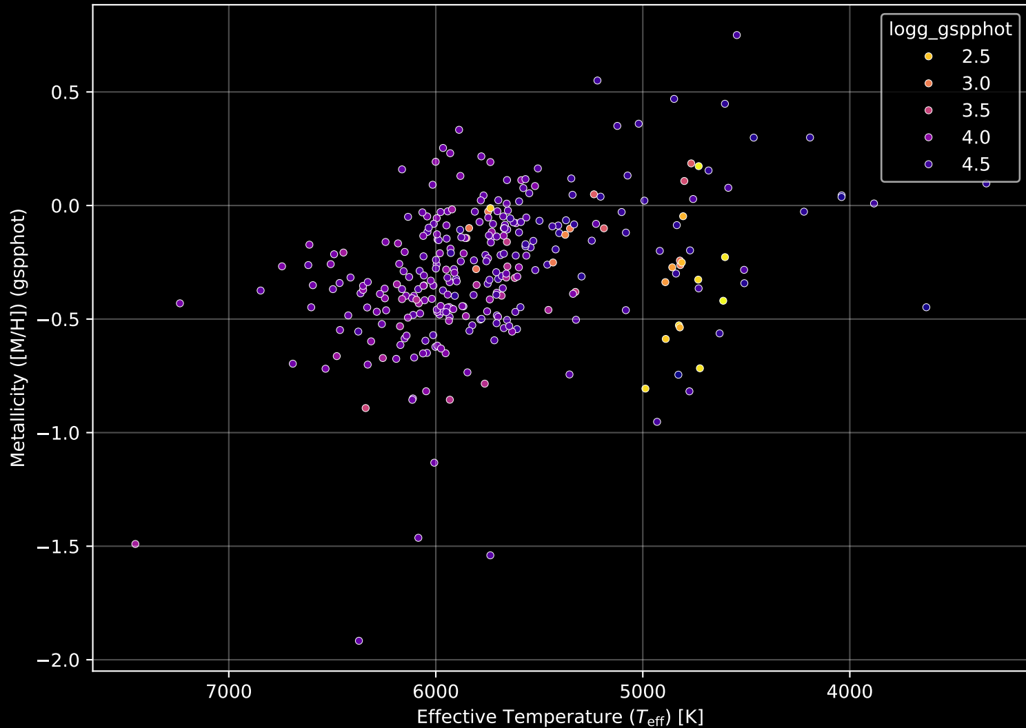
GALAH DR4 Field: [457] Stellar Population Parameters (n= 309)
