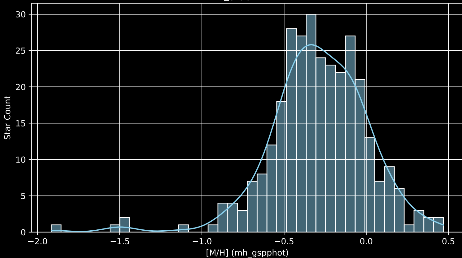
GALAH DR4 Field: [457] [M/H] (mh_gspphot) (n= 307)
