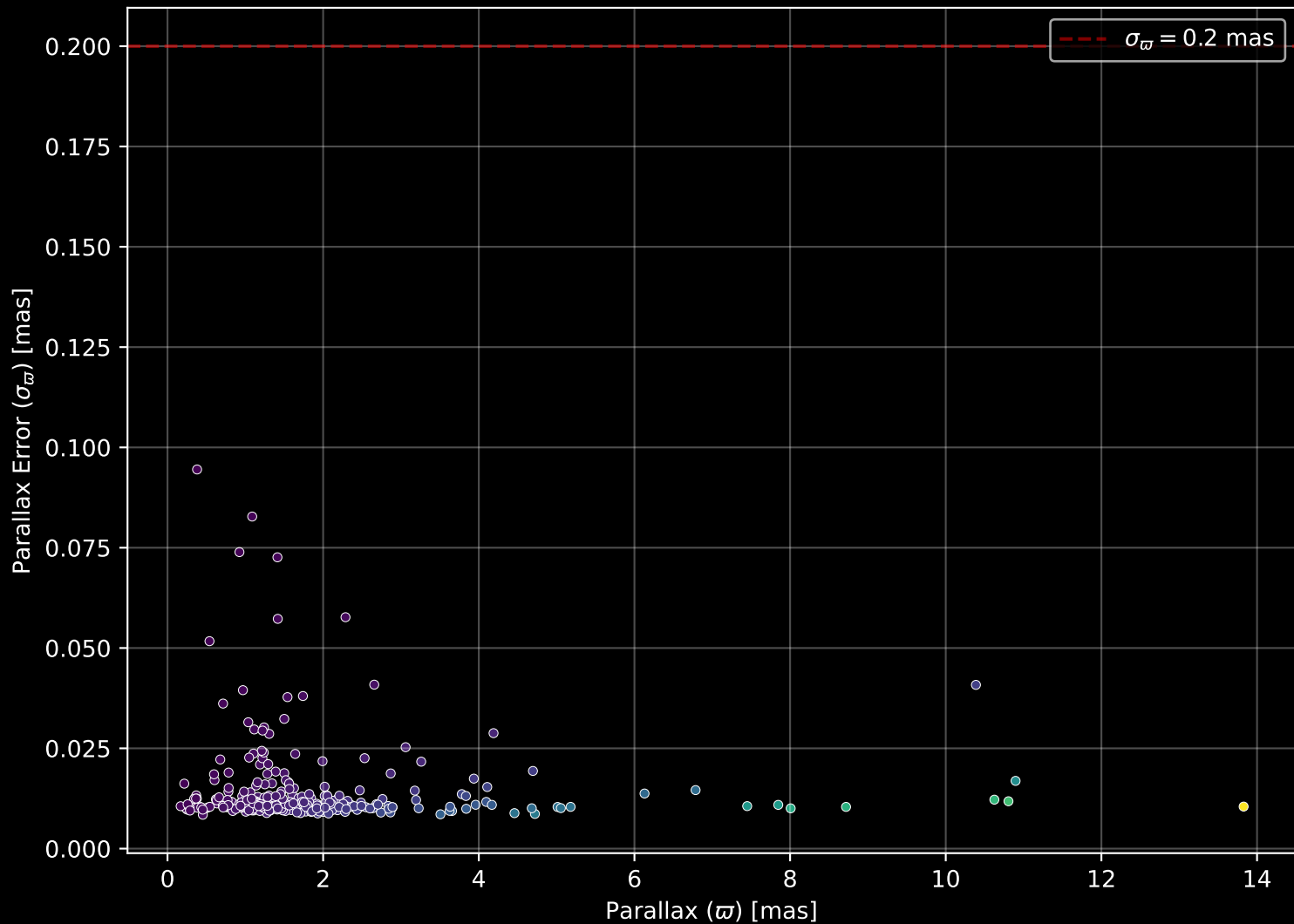
GALAH DR4 Field: [457] Parallax Quality (n= 309)
